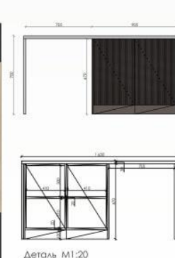
Деталь M1:20
