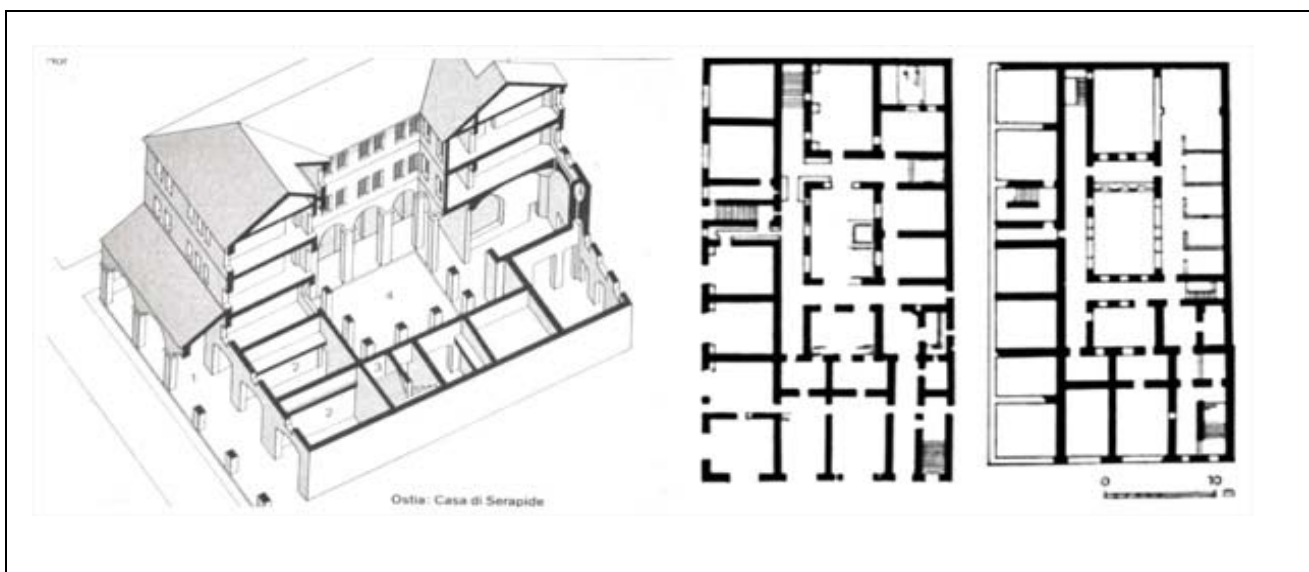
Рис.1.3.1. Давньоримська інсула.
